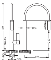
Monomando fregadero vertical con rociador extraíble
