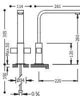
Bimando fregadero vertical caño de 35x15 mm.
