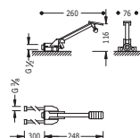
Grifo de pedal Mezclador. Presionando el pedal aumenta progresivamente la temperatura del agua, siempre con un caudal constante.
