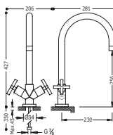
Bimando fregadero vertical
