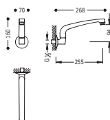
Caño fundido giratorio de 20,4 cm. (pared)
