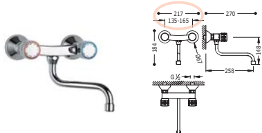
Grupo fregadero pared
