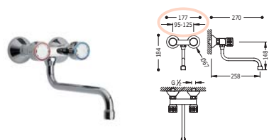
Grupo fregadero pared Distancia a pared de 260 mm.
