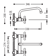
Grupo fregadero pared Distancia a pared de 330 mm.
