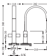
Bimando fregadero vertical caño 35x15 mm. con aireador rectangular oculto
