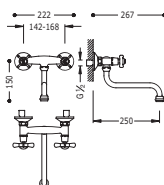
Grupo fregadero pared Distancia a pared de 250 mm.
