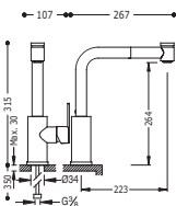
Monomando fregadero vertical con ducha extraíble (2 funciones)
