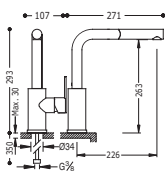
Monomando fregadero vertical con ducha extraíble
