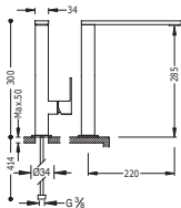
Monomando fregadero vertical caño de 34x10 mm.
