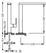
Monomando fregadero vertical caño de 34x15 mm.
