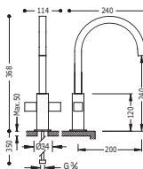
Bimando fregadero vertical caño de 22x22 mm.
