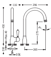
Monomando fregadera vertical con rociador extraíble
