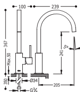
Monomando fregadero vertical caño de 22x22 mm.
